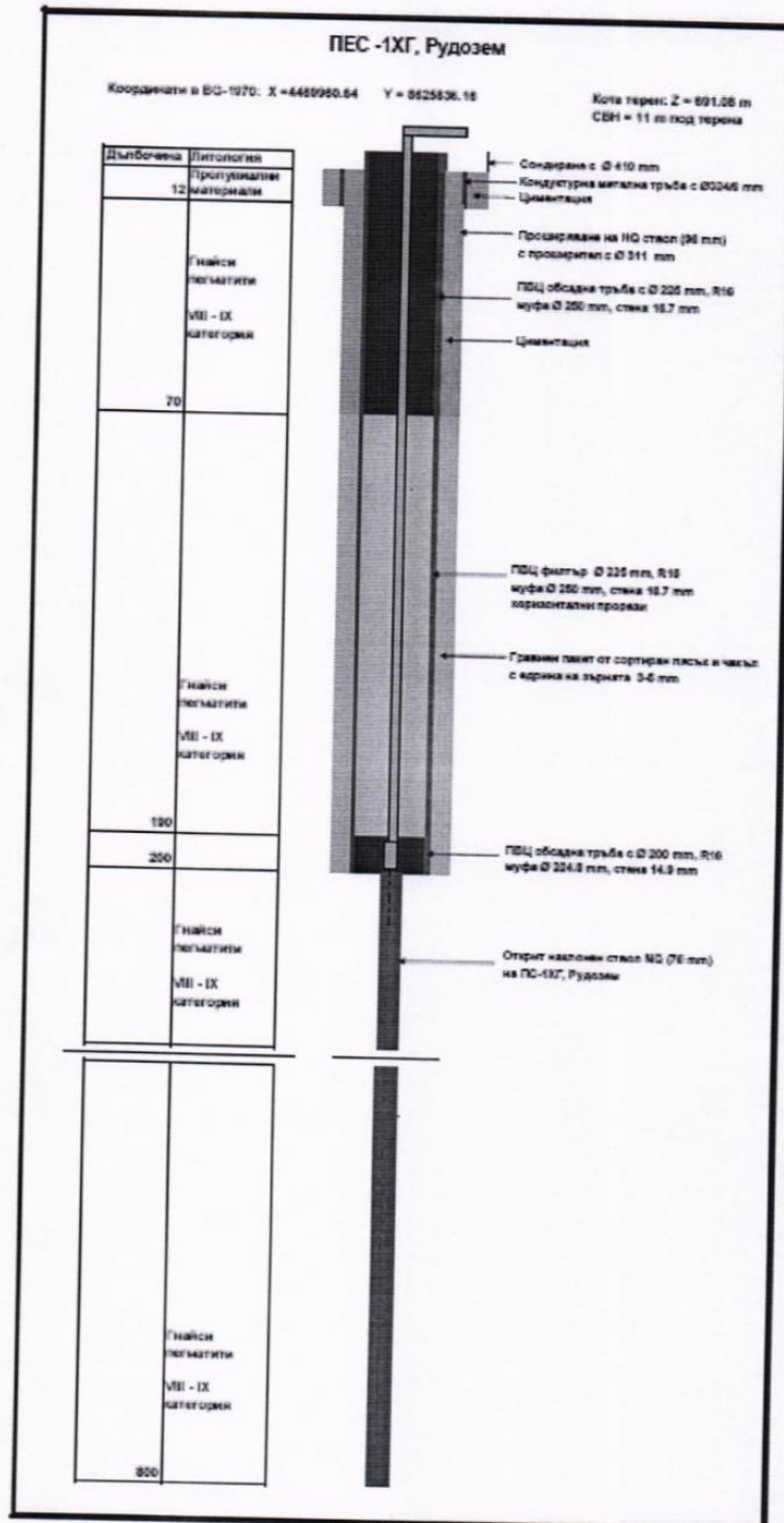
Фиг. 2. Проектна конструкция на ПЕС-1ХГ, Рудозем
